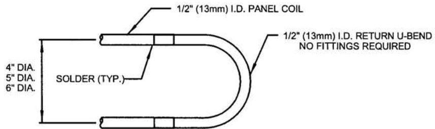
RETURN U-BEND (B)
